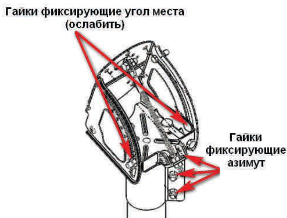
Рисунок 33 – Гайки, фиксирующие угол места и азимут
