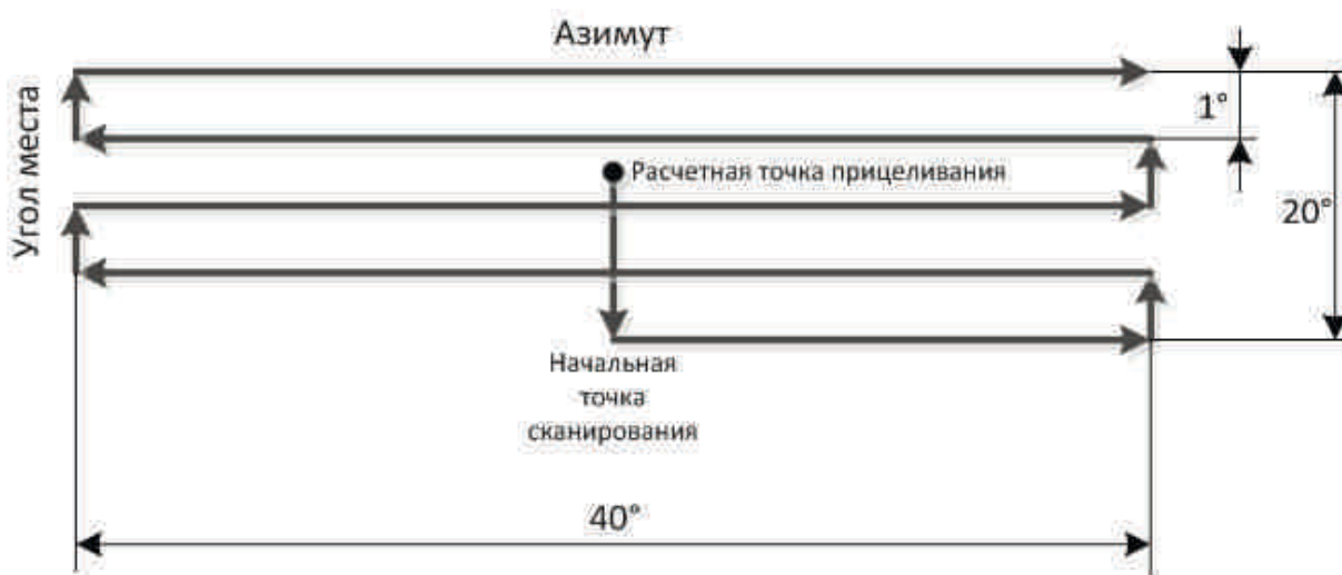
Рисунок 36 – Нарезка линий горизонта
