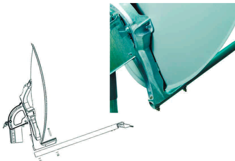
Рисунок 25 – Крепление штанги
