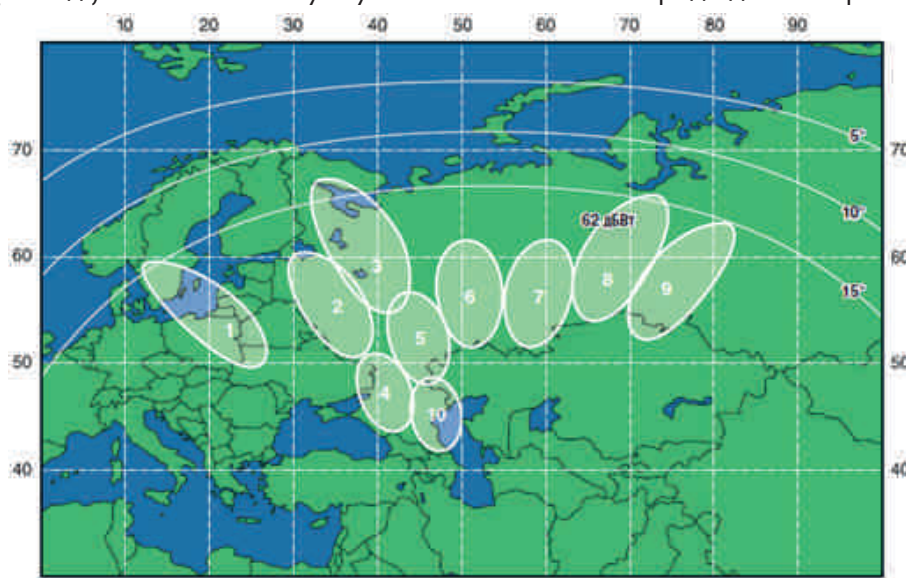
Рисунок 3 – Зона покрытия лучей Ка диапазона «Экспресс АМ6»
