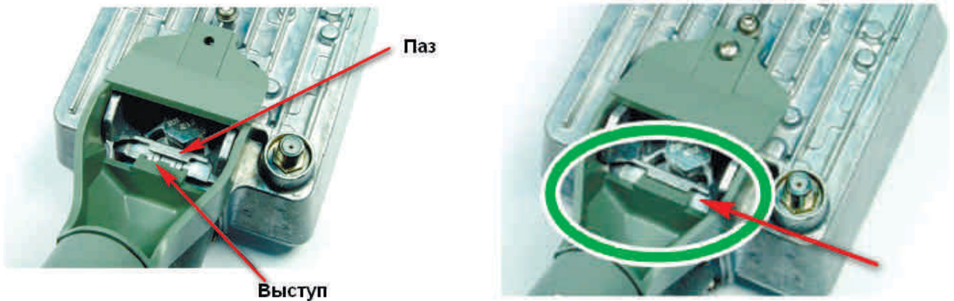
Рисунок 27 – Фиксация приемопередатчика
